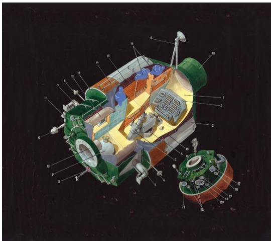
Entwurf für das Technikmodul der Raumstation Mir (1980) © Archiv Galina Balaschowa
